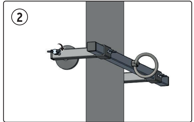
An die Wand klemmen und fixieren
