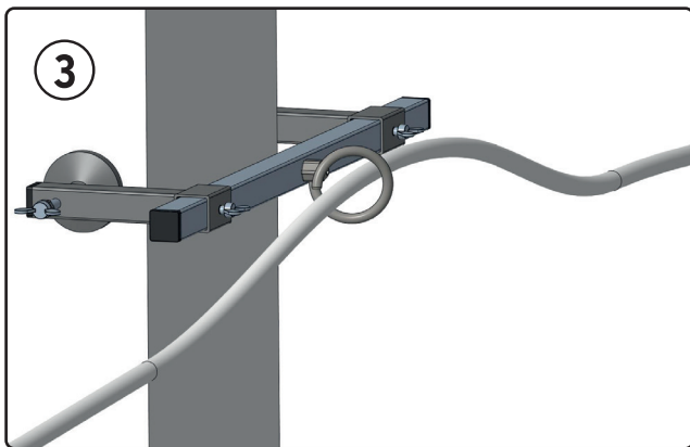
Rohr durch Führungsring ziehen
