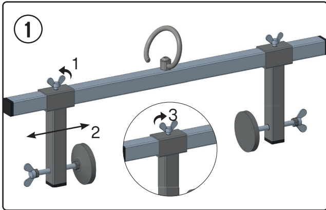
Verstelleinheit verschieben und fixieren
