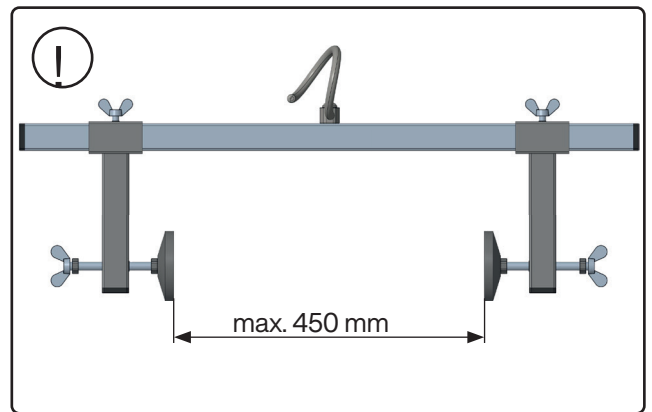
Die maximale Mauerdicke beachten
