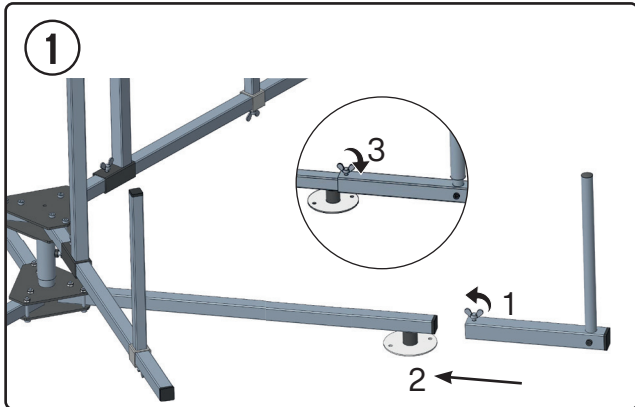
Adapter an Haspel befestigen
