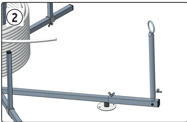
Adapter für Rohrführungsauge
