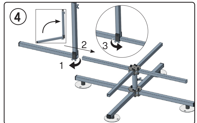
Führungsstange mit Verlängerung aufschieben und befestigen.
