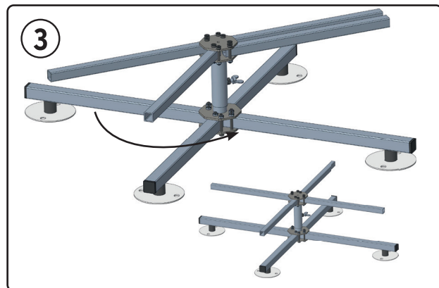
Ausleger um 45° ausbreiten.
