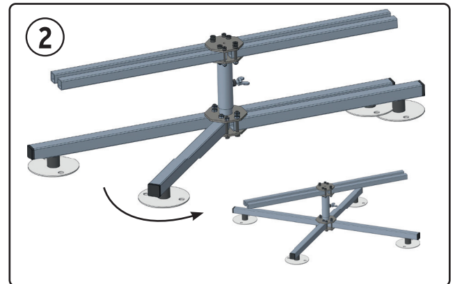
Standfüße um 45° ausbreiten.
