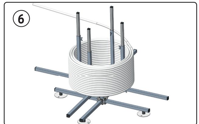
Rohrcoil aufsetzen und Rohrende abwickeln.
